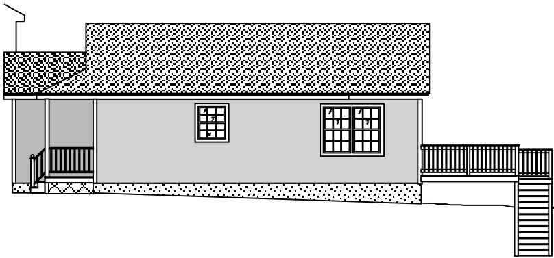
right elevation
