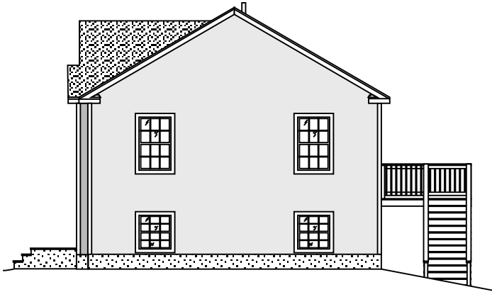
right elevation
