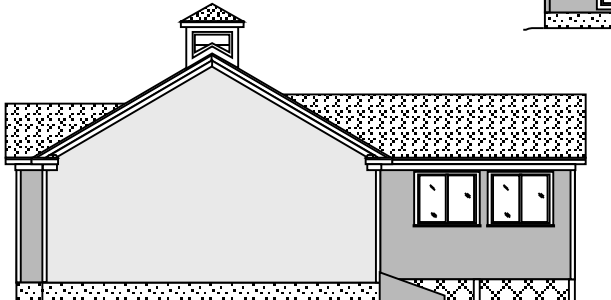
right elevation
