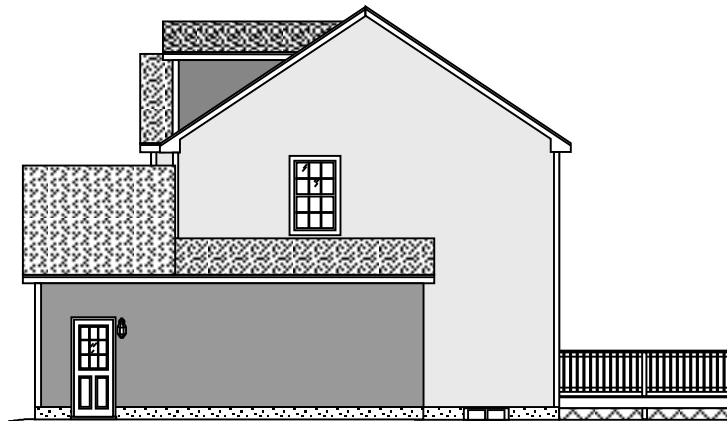
right elevation
