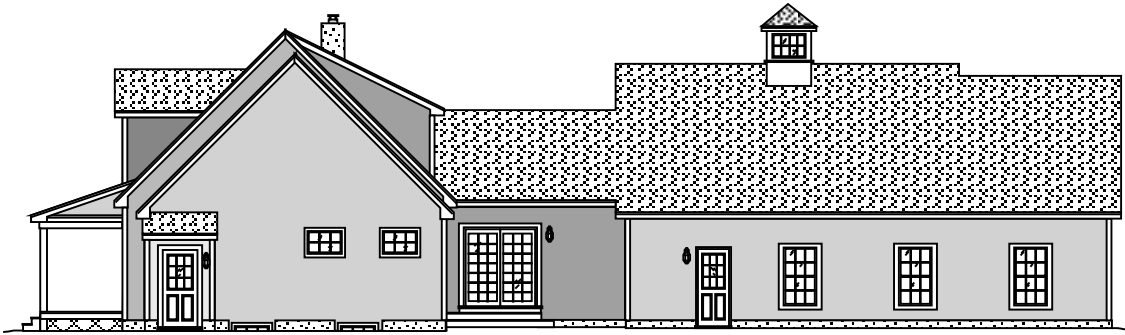
right elevation
