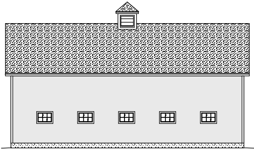
right elevation
