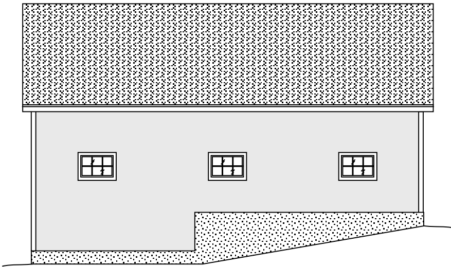
right elevation
