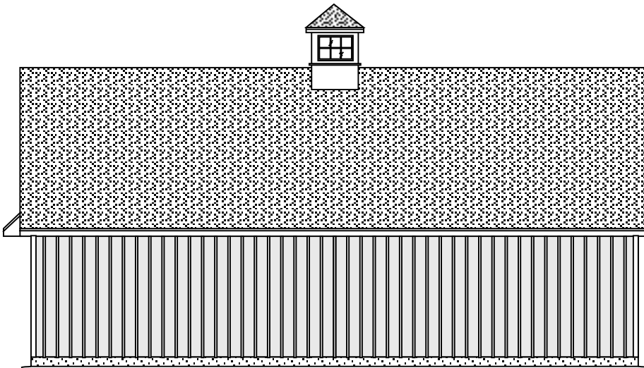
right elevation
